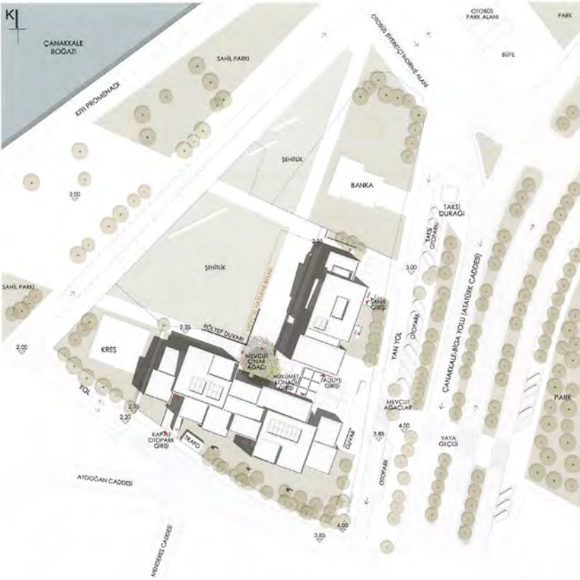
VAZİYET PLANI
